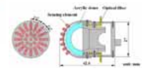
触覚センサ(3軸力検知)
